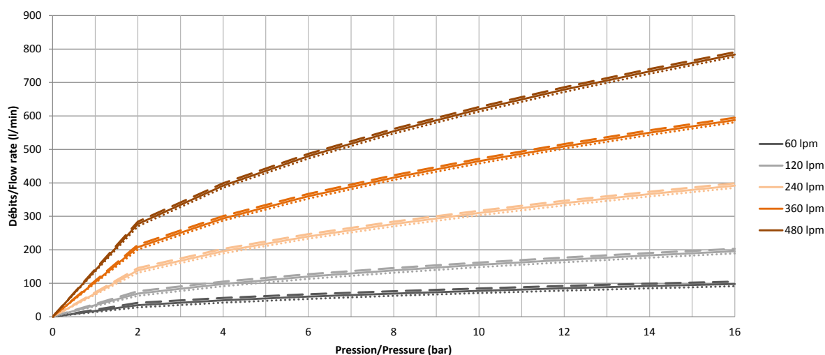
COURBE DÉBITS / PRESSIONS
